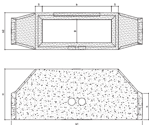
Pozzetto ENEL a 90°
