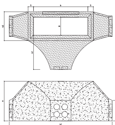
Pozzetto ENEL a 3 vie
